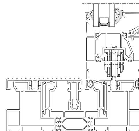
heroal S 65 met barrièrevrije dorpel, zonder extra isolatie en met standaard afdichtingen, doorsnede-aanzicht
