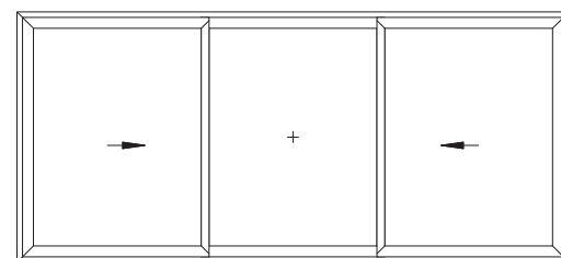
Beslagschema K: 2 schuifvleugels, 1 vaste vleugel
