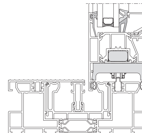
heroal S 65 HI met barrièrevrije dorpel, met extra isolatie en met HI afdichtingen, doorsnede-aanzicht
