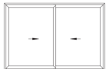
Beslagschema D: 2 schuifvleugels
