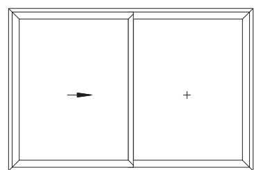
Beslagschema A (links): 1 schuifvleugel, 1 vaste vleugel
