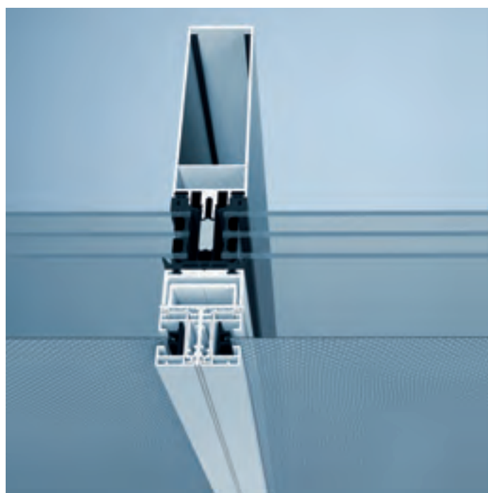
Gedeeltelijk in de vliesgevel geïntegreerd zonweringssysteem heroal VS Z CS
