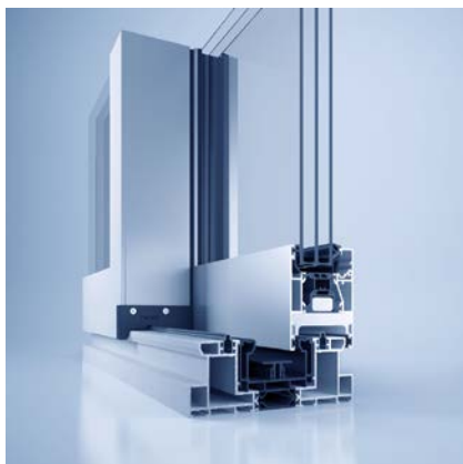
[heroal S 65]
