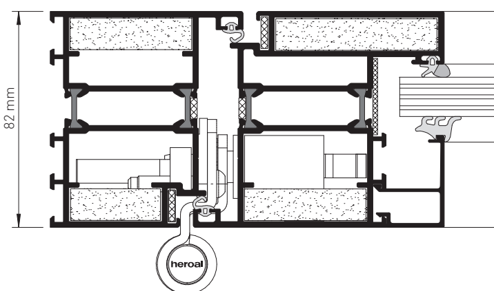
heroyal D 82 FP, Schnittdarstellung, Maßstab 1:2
