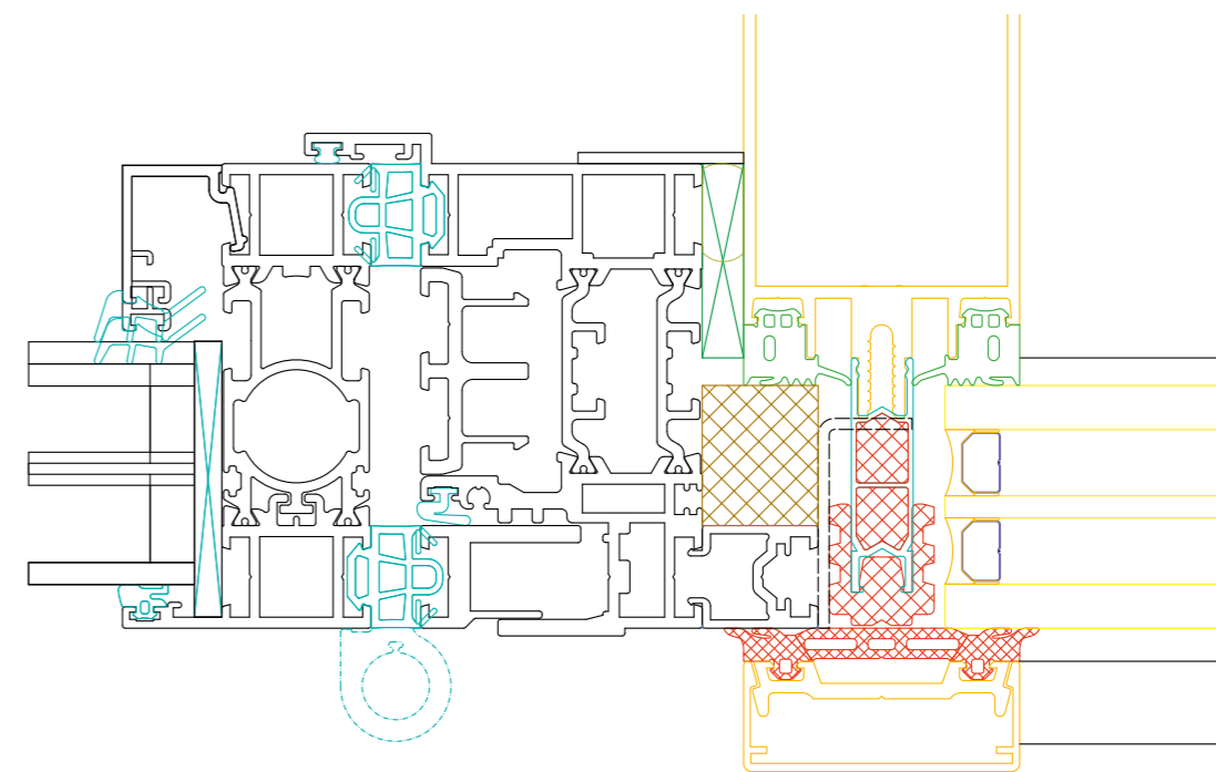
Fassadensystem heroal C 50 HI mit Solarlux Glas-Faltwand Highline
