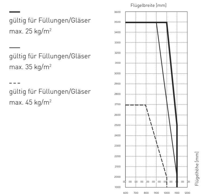
Solarlux Glas-Faltwand Highline, Flügelgrößen (Maße inkl. Rahmenanteil)
