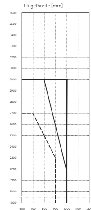
Solarlux Glas-Faltwand Ecoline, Flügelgrößen (Maße inkl. Rahmenanteil)
